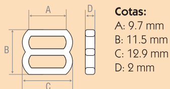
C11T Corredera de 11 mm
