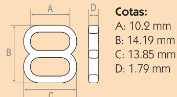
NC11T Corredera de 11 mm bretel grueso
