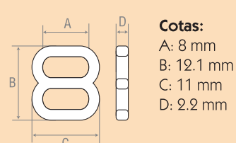
C8T Corredera de 8 mm
