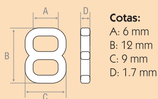
C6T Corredera de 6 mm
